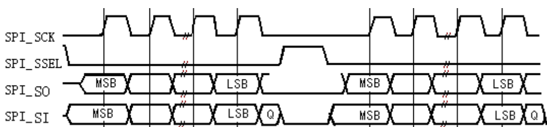
图表 5 SPI 通讯时序图
