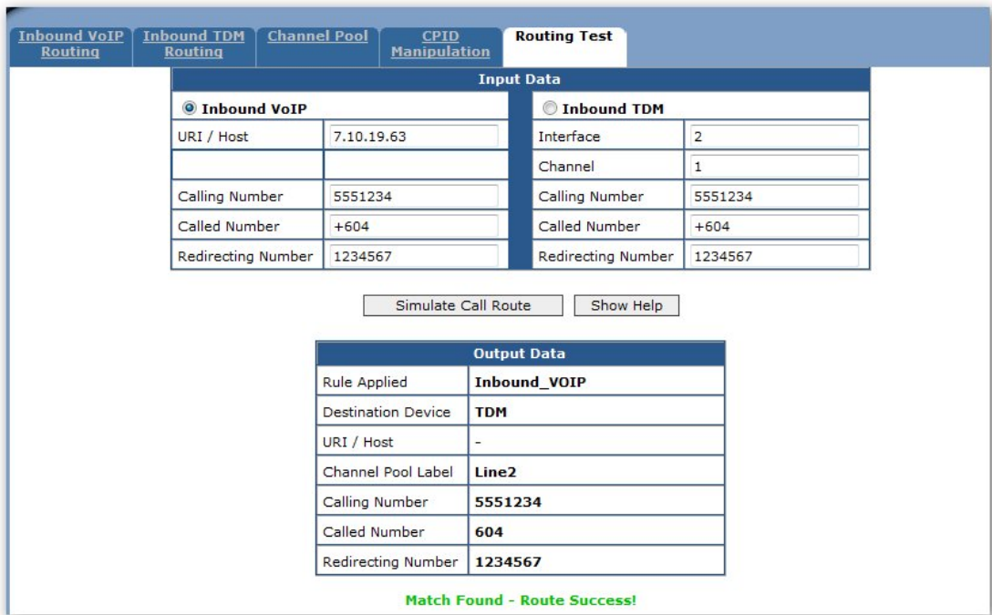
图 6.3 验证 VOIP 呼叫路由
