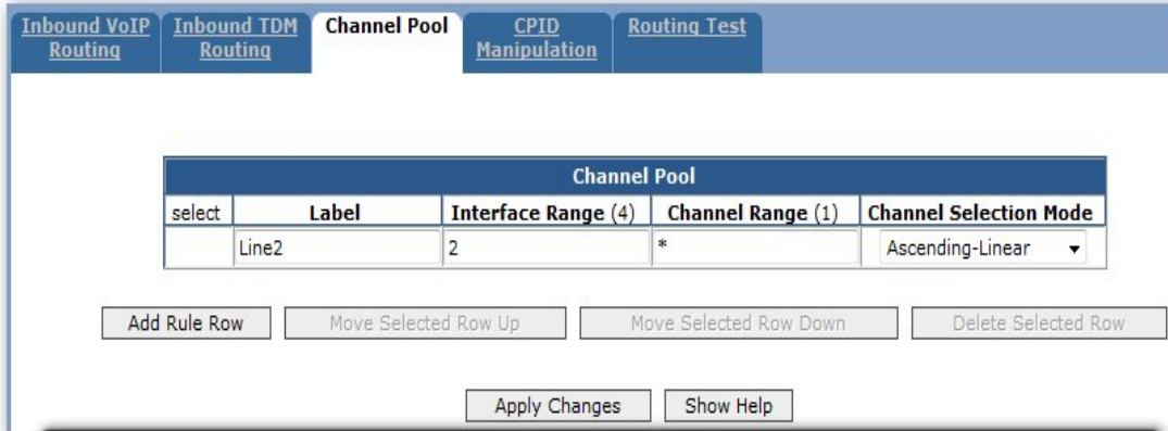
图 4.1 为 DMG 的第二个电话接口设定号码
